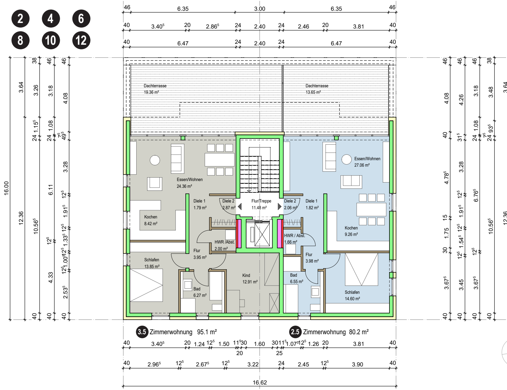
GRUNDRISS ATTIKAGESCHOSS (3- und 4-geschossiges Gebäude)
