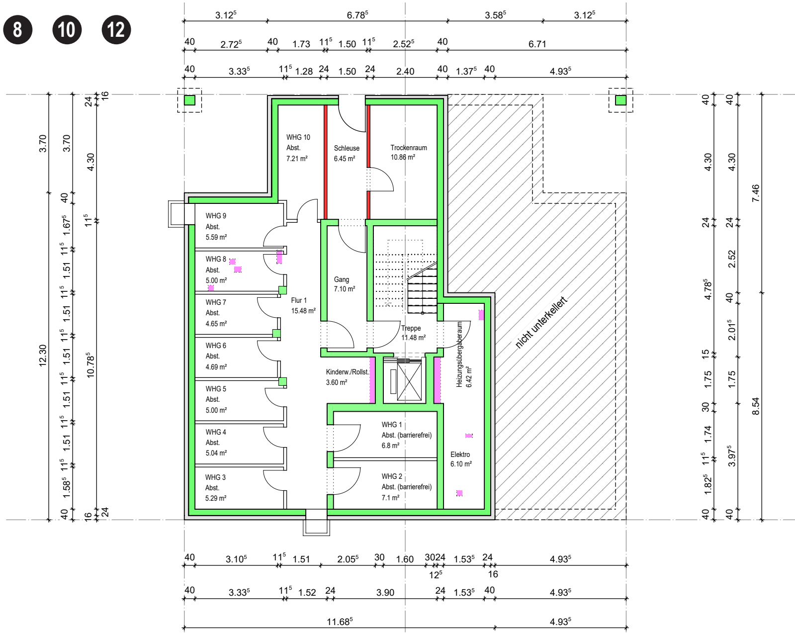
GRUNDRISS UNTERGESCHOSS (4-geschossig)
